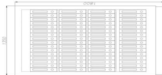
HAMBURG 45006 Art. Nr. 45006 # 150/1350/317 64 Ordner in vier Reihen
