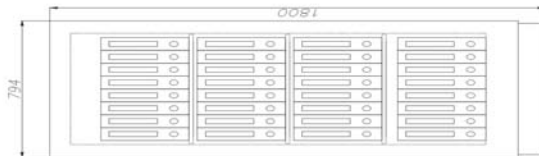
HAMBURG 45005 Art. Nr. 45005 # 150/794/317 32 Ordner in vier Reihen
