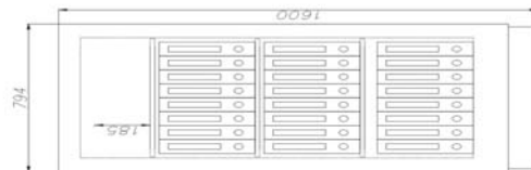
HAMBURG 45004 Art. Nr. 45004 # 150/794/317 24 Ordner in drei Reihen Fachböden 185 hoch
