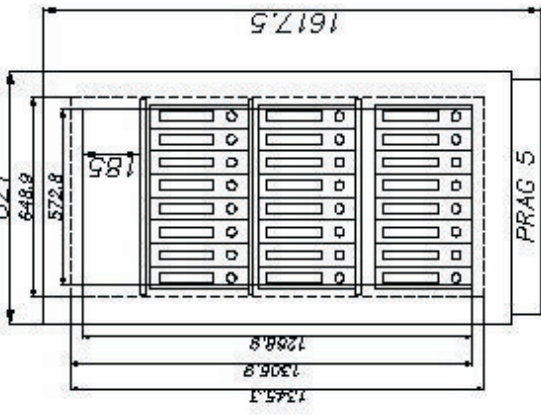
AM 1617.5x821x573 IM 1306.9x648.9x331 24 Ordner in drei Reihen Fachboden 185 hoch
