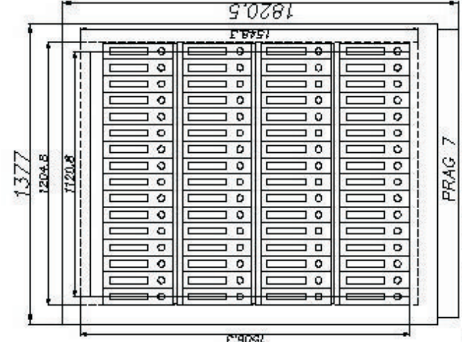
PRAG 7 AM 1820,5 x 1377 x 573 IM 1506,3 x 1204,8 x 331 64 Ordner in vier Reihen
