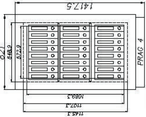
AM 1417.5x821x573 IM 1107.3x648.9x331 24 Ordner in drei Reihen
