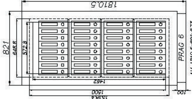
PRAG 6 AM 1810,5x821x573 IM 1500x648,8x331 32 Ordner in vier Reihen
